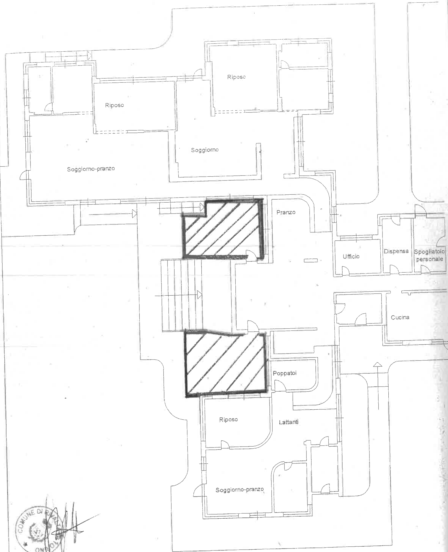
Asilo Nido, ex "Scuola Materna Sangone" - Piano Terreno, Scala 1:200
